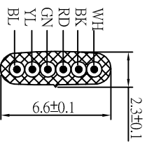
SECTION A-A T0060
